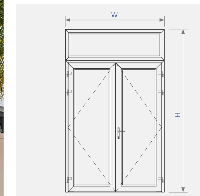
Sơ đồ lắp ráp cửa đi mở quay 2 cánh hệ 93XFA PRO
