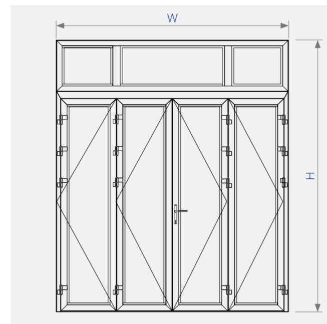
Sơ đồ lắp ráp cửa đi mở quay 4 cánh hệ XFA55
