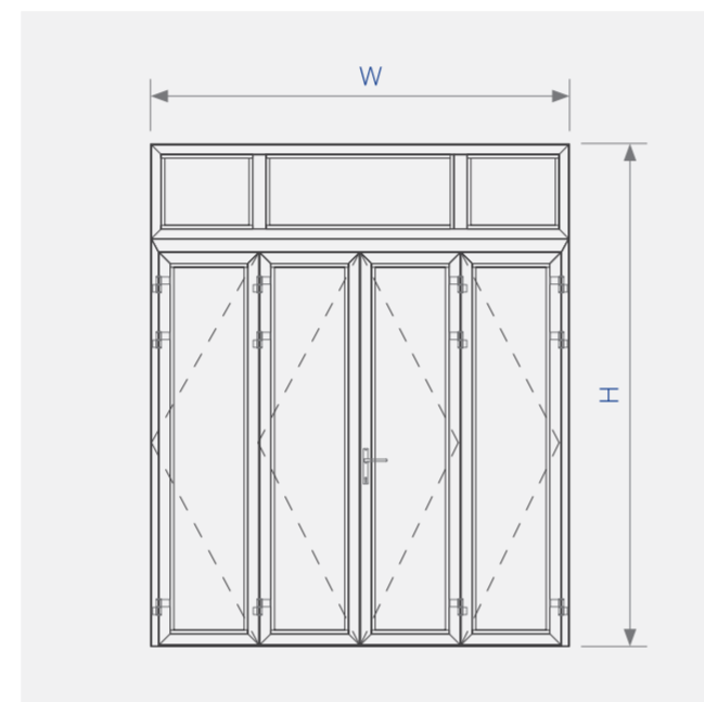
Sơ đồ lắp ráp cửa đi mở quay 4 cánh hệ 93XFA PRO
