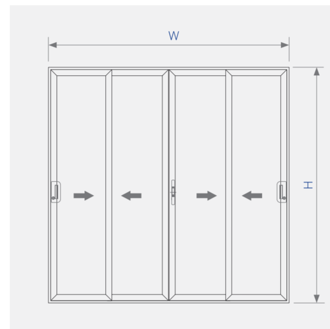
Sơ đồ lắp ráp cửa đi lùa 4 cánh hệ 93XFA PRO
