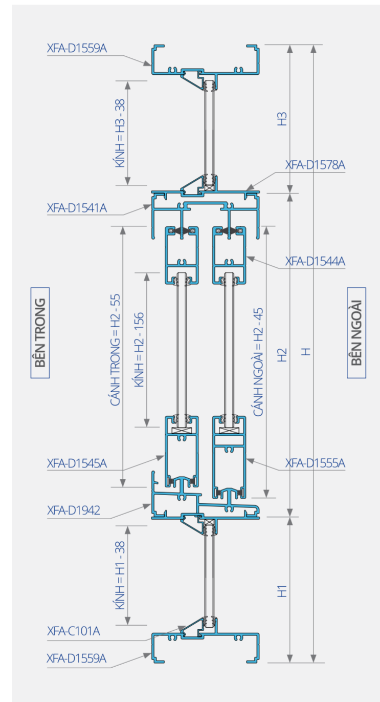
Sơ đồ lắp ráp cửa sổ lùa 2 cánh hệ XFA93
