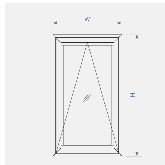
Sơ đồ lắp ráp cửa sổ mở hất 1 cánh hệ XFA55
