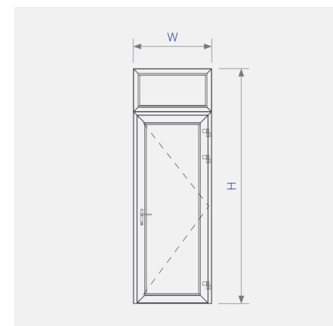
Sơ đồ lắp ráp cửa đi mở quay 1 cánh hệ 93XFA PRO
