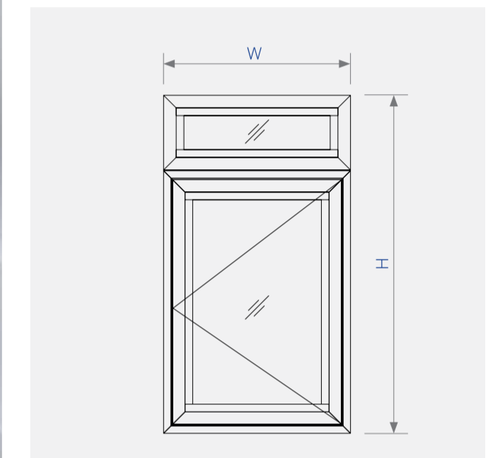
Sơ đồ lắp ráp cửa sổ mở quay 1 cánh hệ XFA1000
