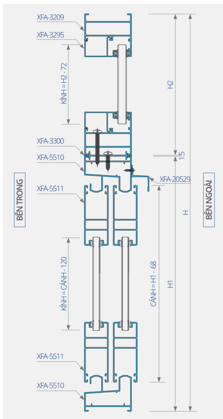
Sơ đồ lắp ráp cửa sổ lùa hệ XFA55
