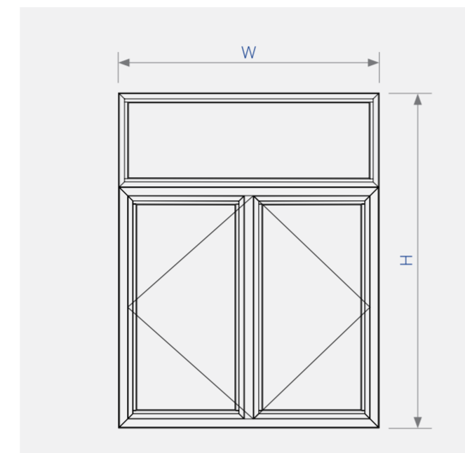
Sơ đồ lắp ráp cửa sổ mở quay 2 cánh hệ XFA55
