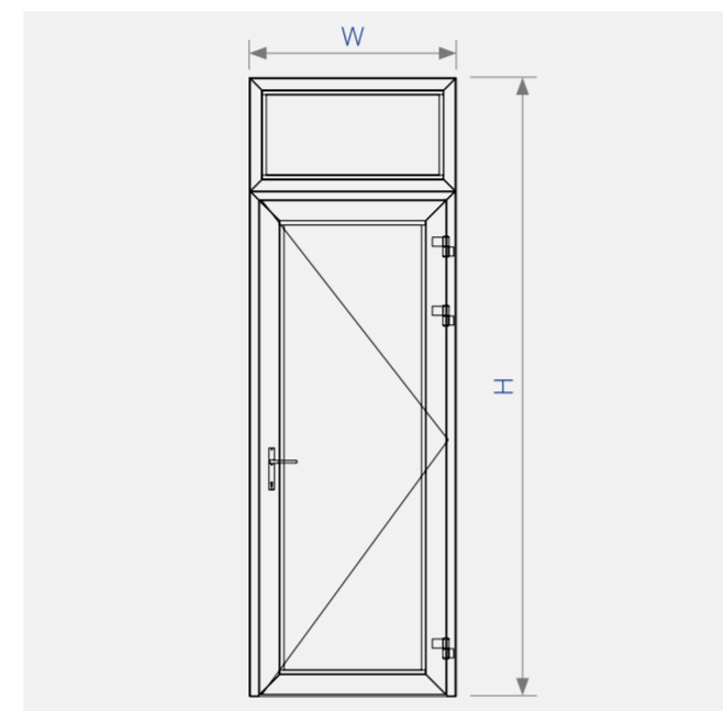
Sơ đồ lắp ráp cửa đi mở quay 1 cánh hệ XFA55
