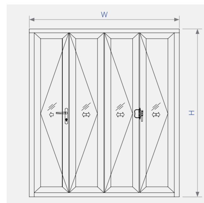
Sơ đồ lắp ráp cửa đi xếp trượt hệ XFA63
