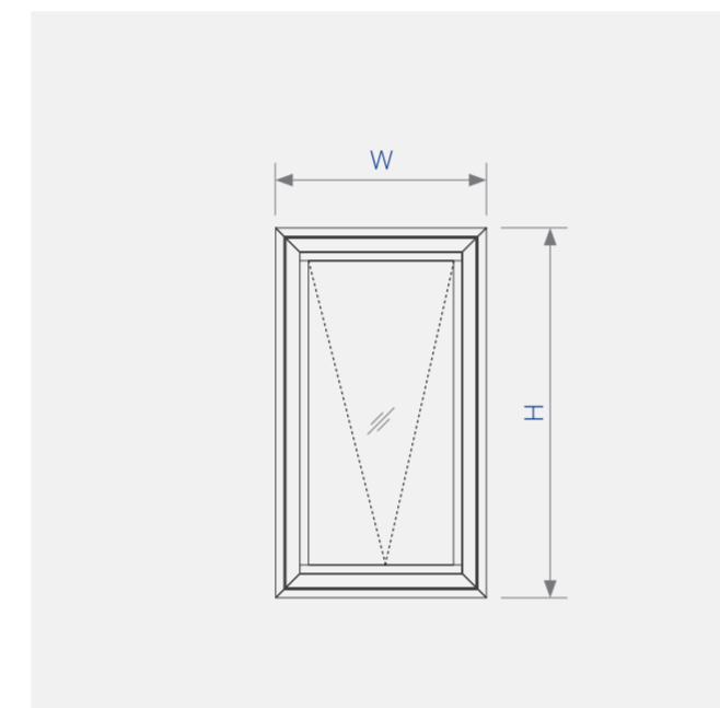
Sơ đồ lắp ráp cửa sổ bật hệ 93XFA PRO
