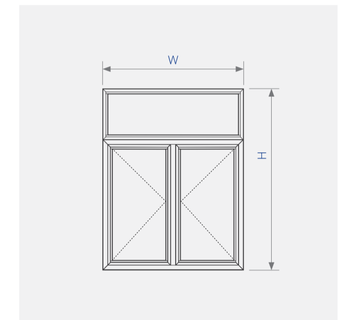
Sơ đồ lắp ráp cửa sổ mở quay 2 cánh hệ 93XFA PRO
